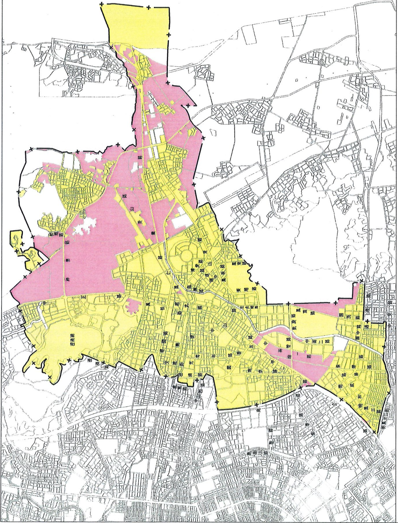
鳳山溪污水區下水道實施地區範圍示意圖
